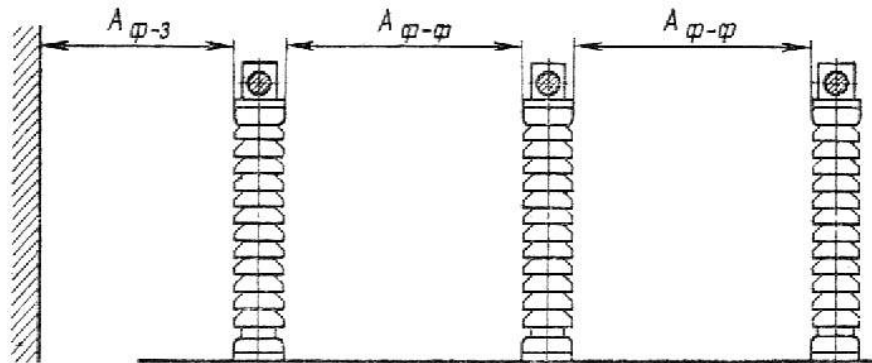
Рис. 4.2.1. Наименьшие расстояния в свету при жестких шинах между токоведущими и заземленными частями ( A_{\phi-з} ) и между токоведущими частями разных фаз ( A_{\phi-\phi} )
